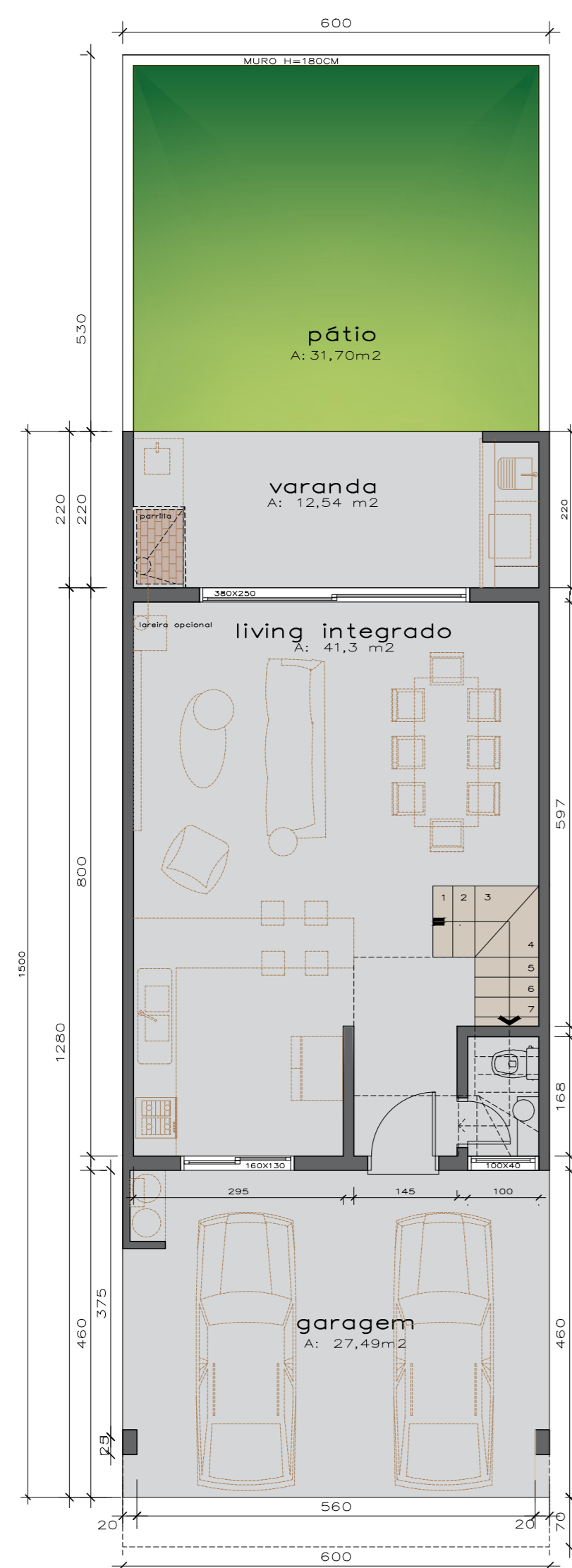
TÉREO A: 90m 2
