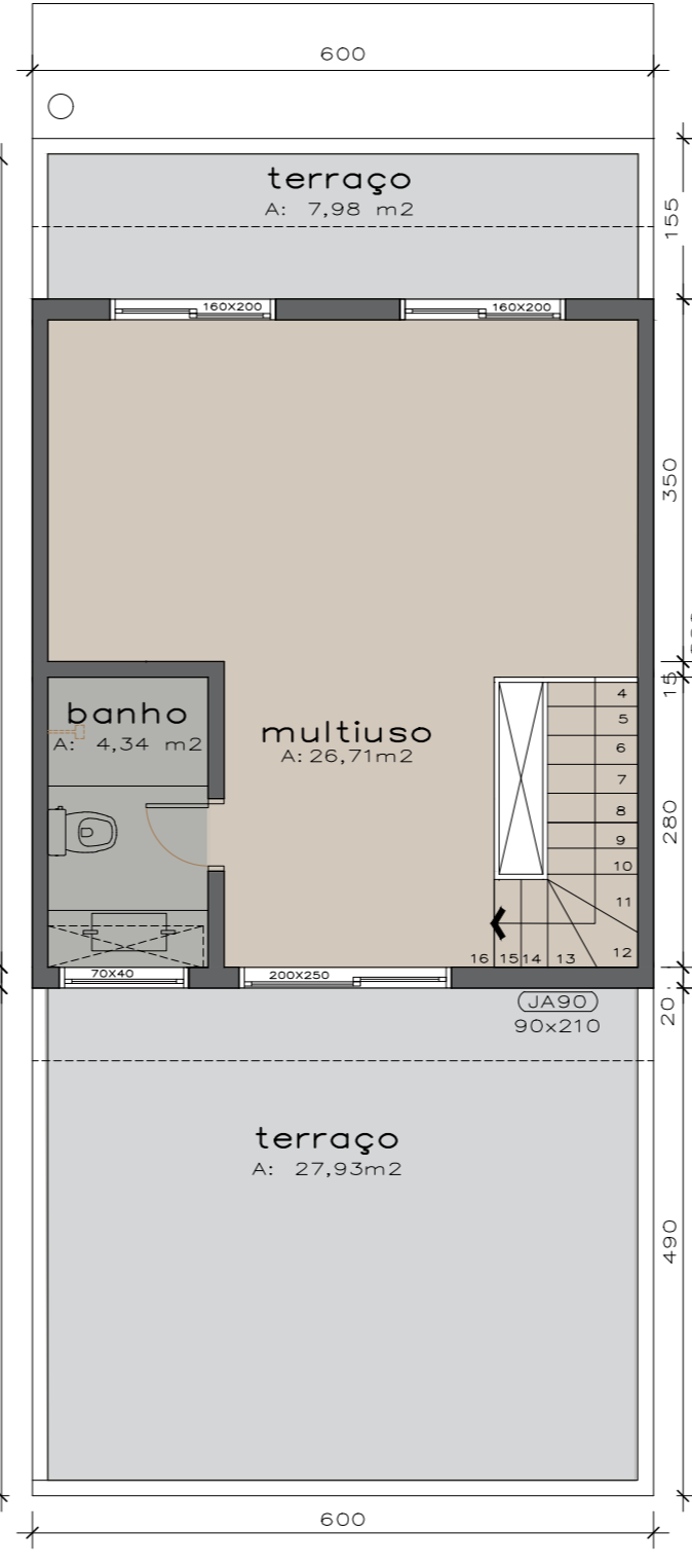
TERCEIRO PAVIMENTO A: 36,00m 2 + 35,9m 2 terraços
