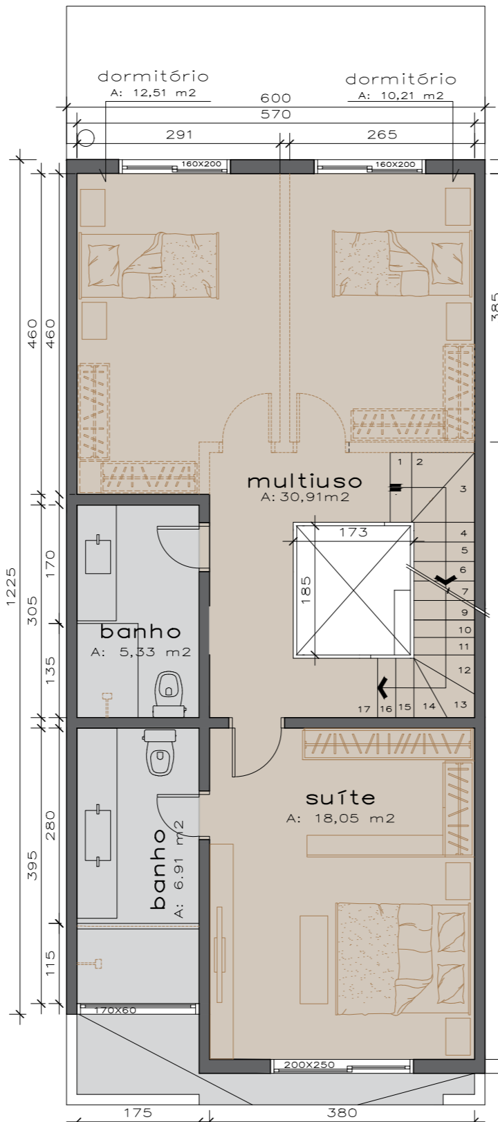
SEGUNDO PAVIMENTO A: 73,60m 2
